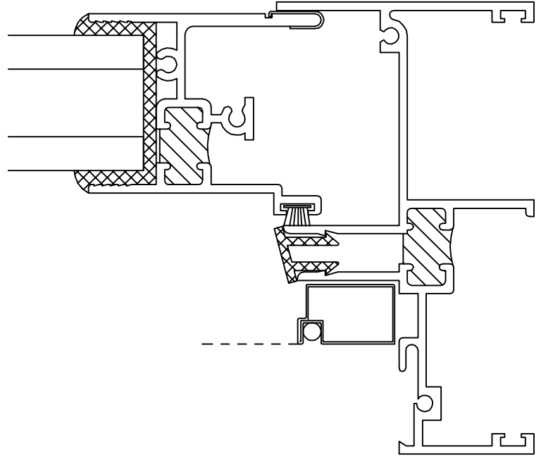
4 SLIDING PANEL JAMB
